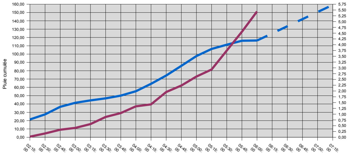
Illustration 3: Évolution du phénomène entre 2 h 15 (début des précipitations) et 7 h 15 (pic de crue) découlant des mesures de la station de Cherchebruit. En rouge les précipitations cumulées (échelle de gauche). En bleu, les hauteurs d'eau (échelle de droite). La station de Cherchebruit a cessé de fonctionner à 6 h 00, le pointillé est une interpolation avec la hauteur constatée en fin de période. Le parallélisme des deux courbes donne une idée de la réactivité du bassin-versant.
