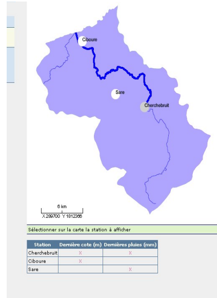
Illustration 2: Le bassin de la Nive et ses trois stations de mesure réglementaires.
